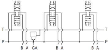
Circuito paralelo con válvula de alivio
