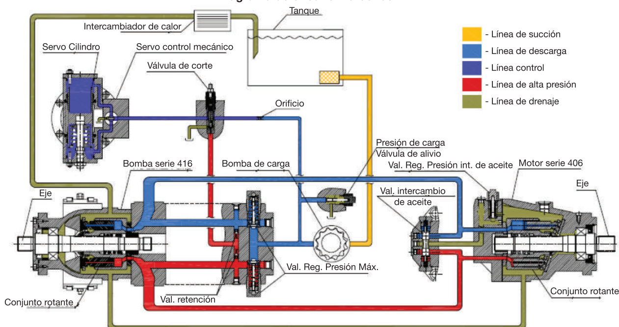
Diagrama de circuito hidráulico
