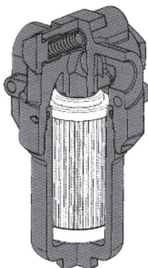
Carcasa
