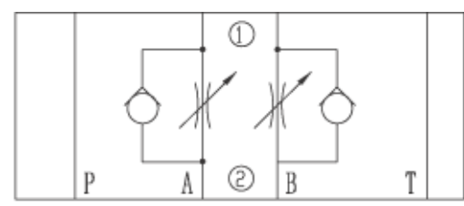
Z2FS6-...-40B/...(meter-out)
