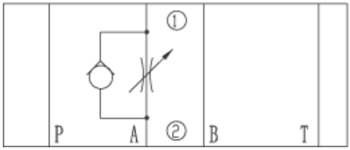
Z2FS 6A-...-40B/...(meter-out)
