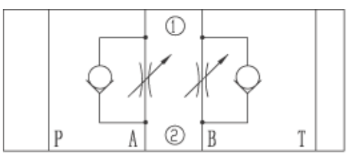
Z2FS6-...-40B/...(meter-in)
